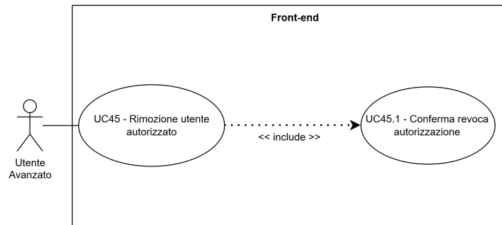
Figure 62: UC45 - Rimozione utente autorizzato
