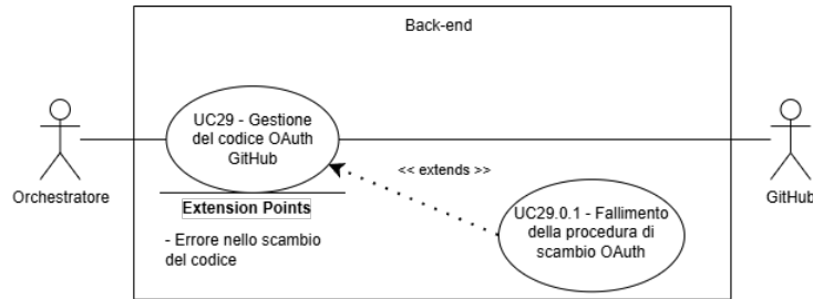
Figure 50: UC29 - Gestione del codice OAuth GitHub
