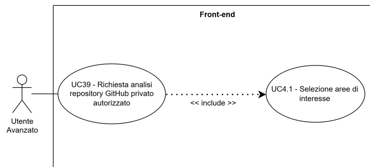
Figure 54: UC39 - Richiesta analisi repository GitHub privato autorizzato
