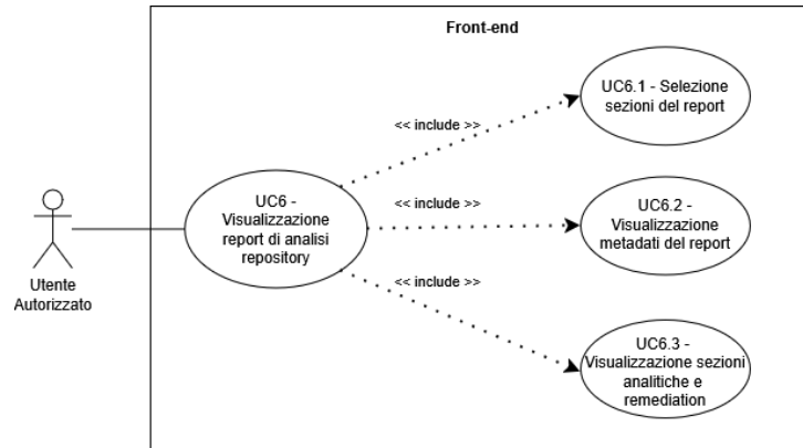
Figure 14: UC6 - Visualizzazione report di analisi
