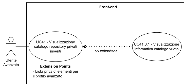
Figure 56: UC41 - Visualizzazione catalogo repository privati inseriti
