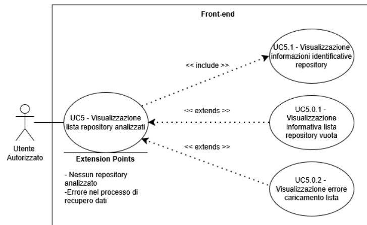
Figure 13: UC5 - Visualizzazione lista repository
