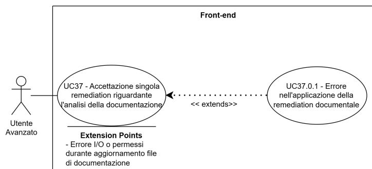
Figure 53: UC37 - Accettazione singola remediation riguardante l'analisi della documentazione
