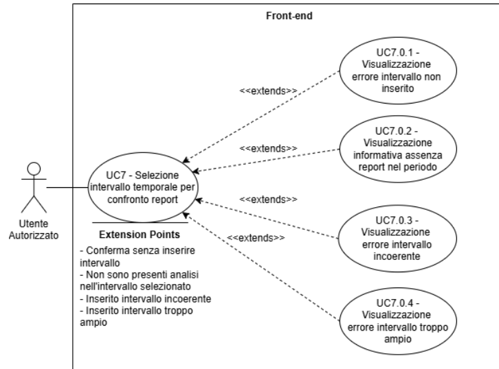
Figure 19: UC7 - Selezione intervallo temporale per confronto report
