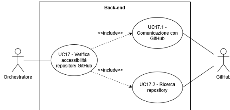
Figure 33: UC17 - Verifica accessibilità repository GitHub
