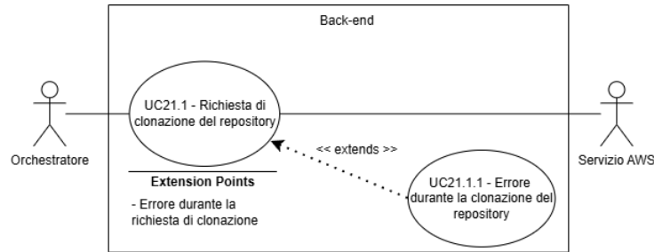
Figure 43: UC21.1 - Richiesta di clonazione del repository
