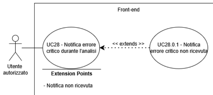
Figure 49: UC28 - Notifica errore critico durante l'analisi
