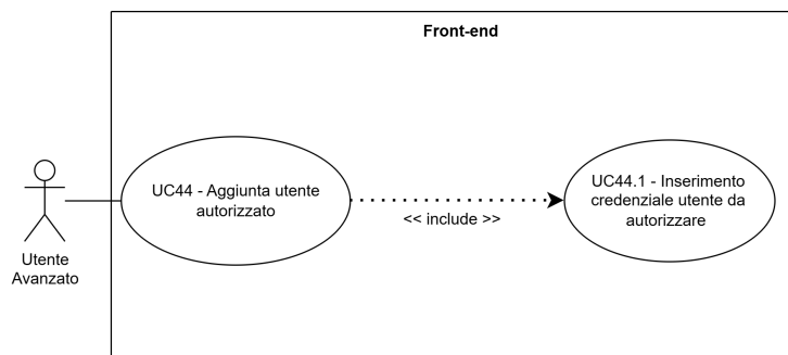
Figure 60: UC44 - Aggiunta utente autorizzato
