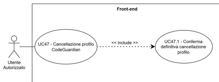
Figure 65: UC47 - Cancellazione profilo CodeGuardian
