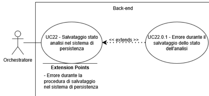
Figure 44: UC22 - Salvataggio stato analisi nel sistema di persistenza
