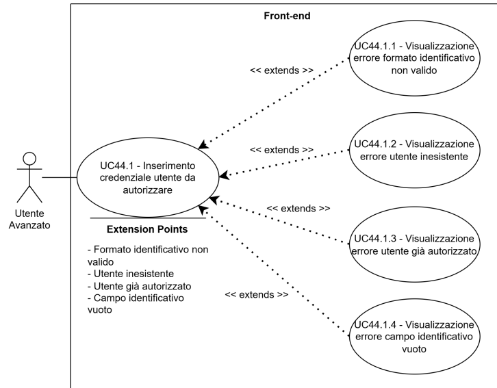
Figure 61: UC44.1 - Inserimento credenziale utente da autorizzare
