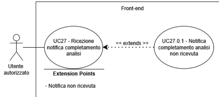
Figure 48: UC27 - Ricezione notifica completamento analisi
