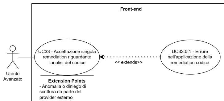
Figure 51: UC33 - Accettazione singola remediation riguardante l'analisi del codice
