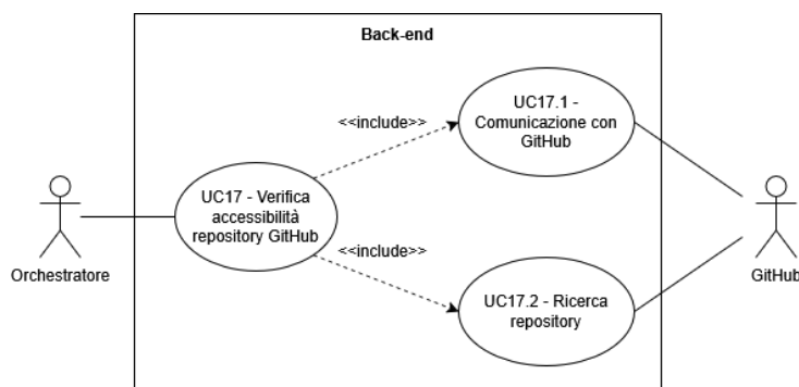
Figure 30: UC17 - Verifica accessibilità repository GitHub
