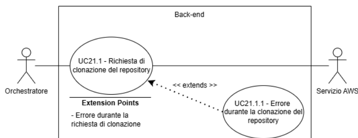
Figure 38: UC21.1 - Richiesta di clonazione del repository
