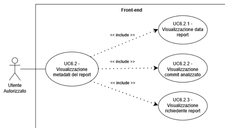
Figure 13: UC6.2 - Visualizzazione metadati del report
