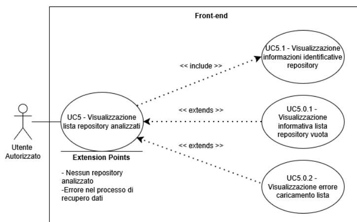
Figure 10: UC5 - Visualizzazione lista repository
