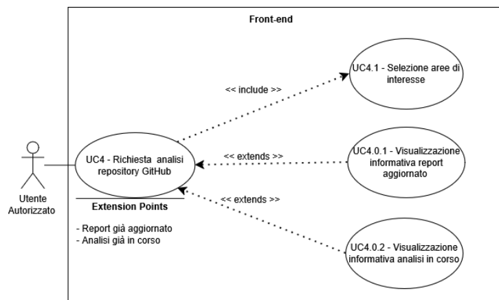
Figure 8: UC4 - Richiesta analisi repository GitHub
