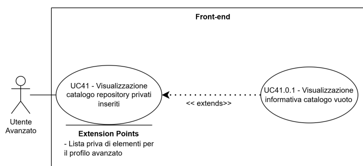
Figure 50: UC41 - Visualizzazione catalogo repository privati inseriti
