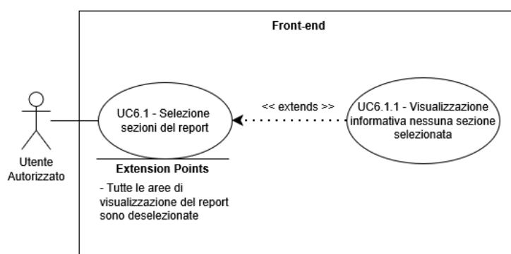
Figure 12: UC6.1 - Selezione sezioni del report
