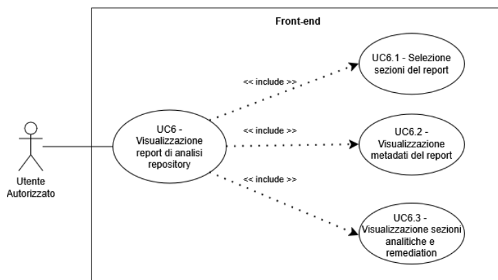
Figure 11: UC6 - Visualizzazione report di analisi
