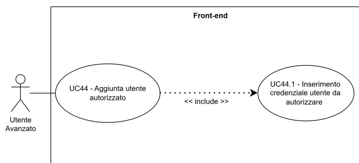
Figure 54: UC44 - Aggiunta utente autorizzato
