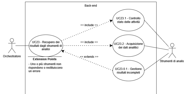
Figure 40: UC23 - Recupero dei risultati dagli strumenti di analisi
