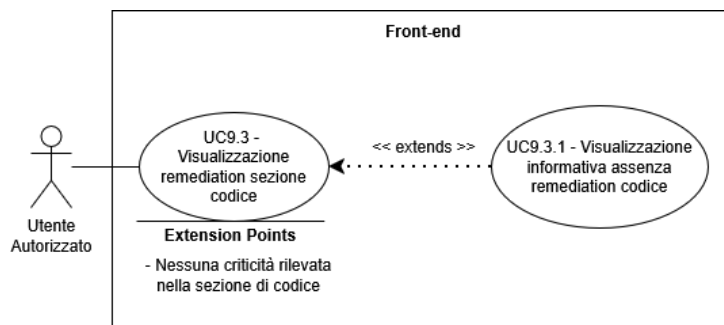
Figure 18: UC9.3 - Visualizzazione remediation sezione codice
