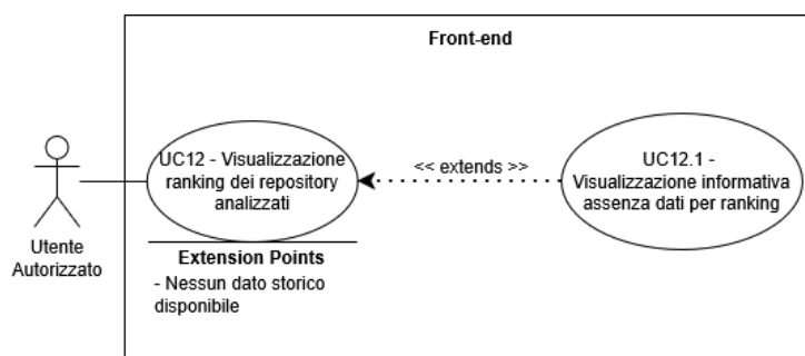
Figure 23: UC12 - Visualizzazione ranking dei repository analizzati
