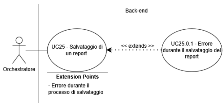
Figure 41: UC25 - Salvataggio di un report
