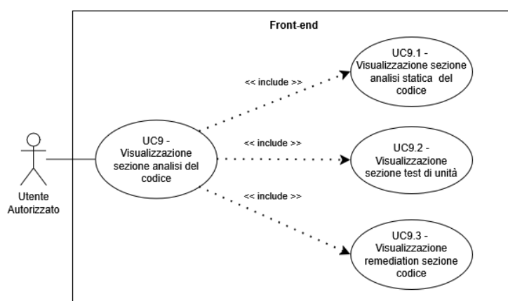
Figure 17: UC9 - Visualizzazione sezione analisi del codice
