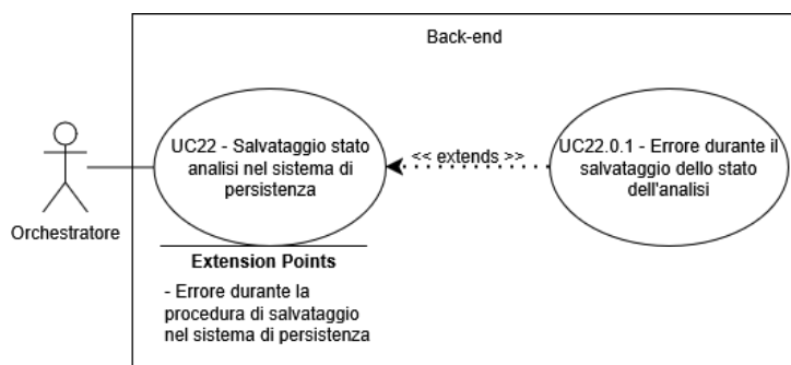
Figure 39: UC22 - Salvataggio stato analisi nel sistema di persistenza
