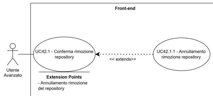
Figure 52: UC42.1 - Conferma rimozione repository
