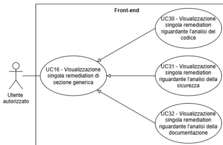
Figure 29: UC16 - Visualizzazione singola remediation di sezione generica
