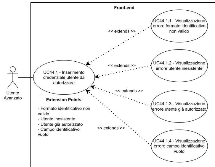
Figure 55: UC44.1 - Inserimento credenziale utente da autorizzare
