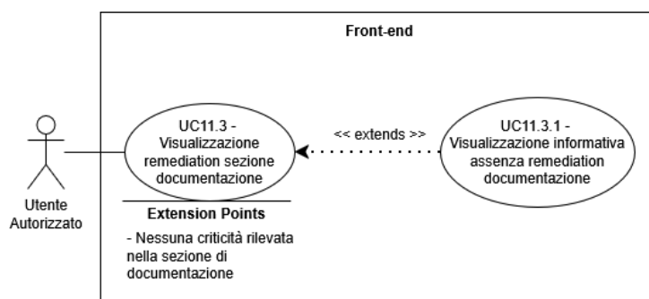
Figure 22: UC11.3 - Visualizzazione remediation sezione documentazione
