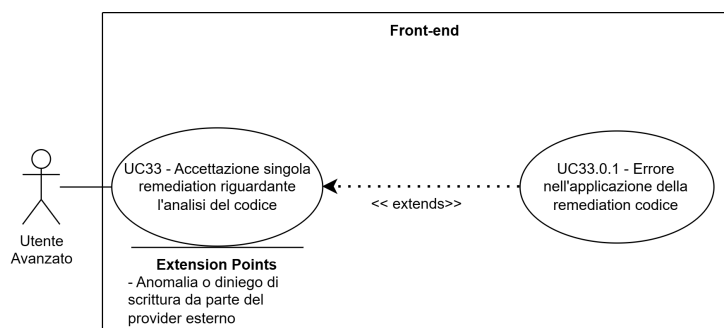
Figure 45: UC33 - Accettazione singola remediation riguardante l'analisi del codice
