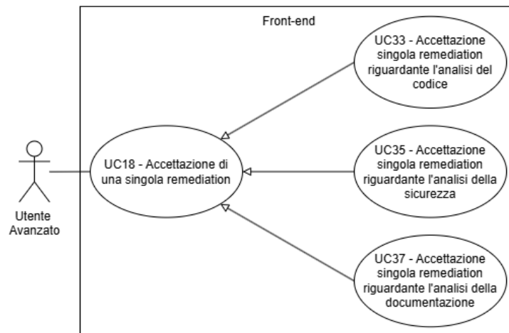
Figure 32: UC18 - Accettazione di una singola remediation
