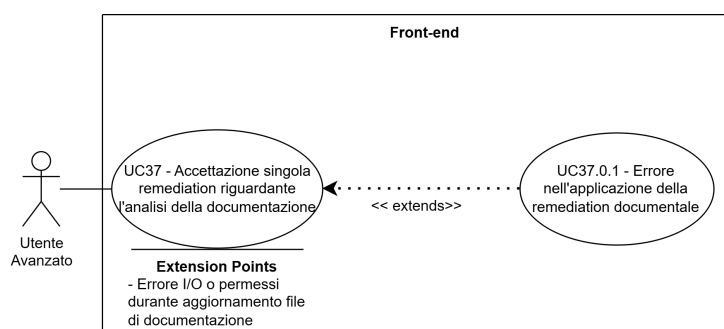
Figure 47: UC37 - Accettazione singola remediation riguardante l'analisi della documentazione
