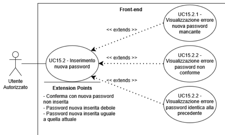
Figure 28: UC15.2 - Inserimento nuova password
