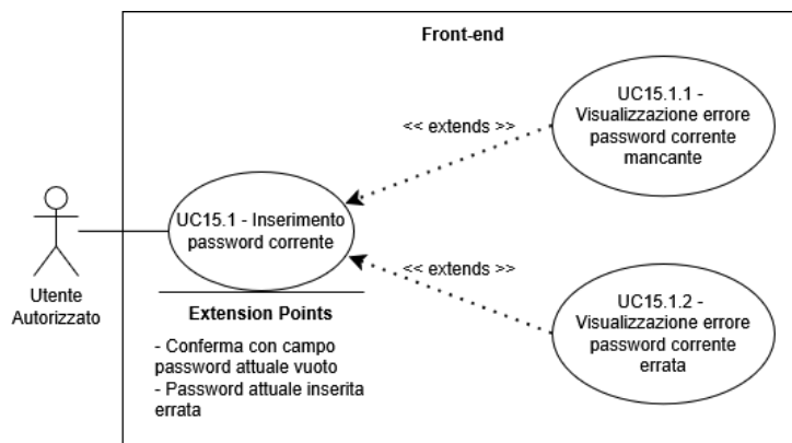
Figure 27: UC15.1 - Inserimento password corrente
