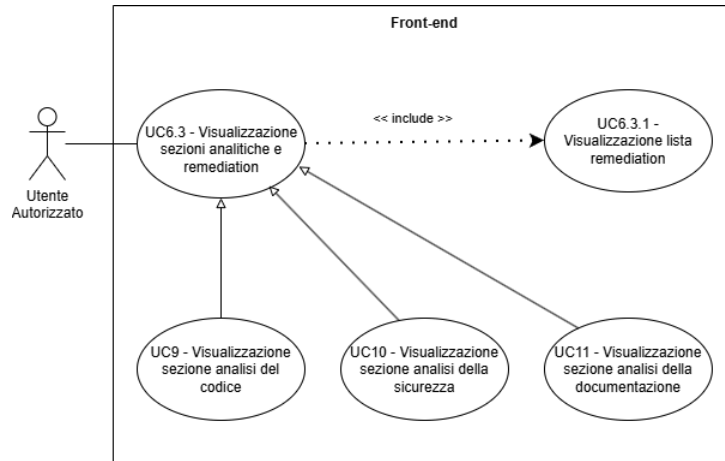
Figure 14: UC6.3 - Visualizzazione sezioni analitiche e remediation
