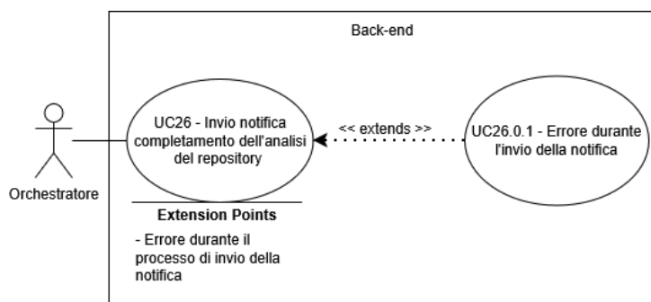
Figure 42: UC26 - Invio notifica completamento dell'analisi del repository
