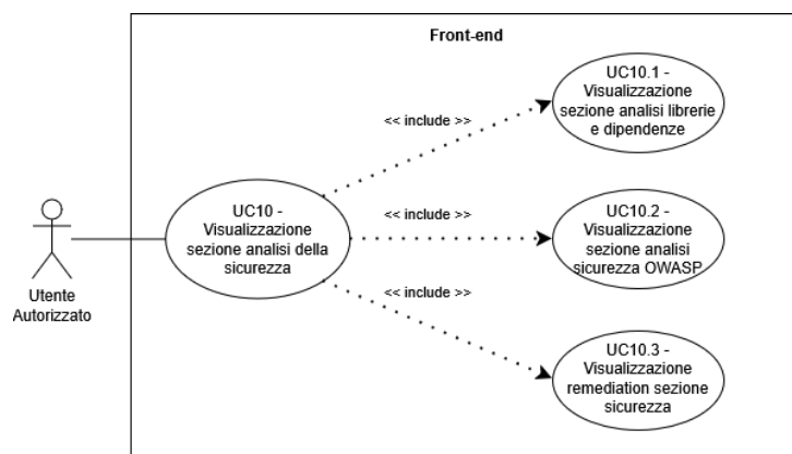
Figure 19: UC10 - Visualizzazione sezione analisi della sicurezza
