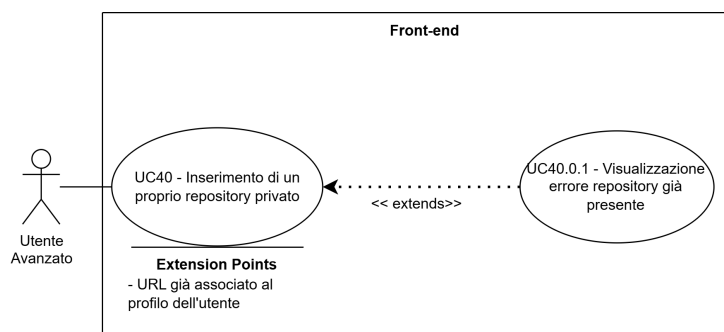
Figure 49: UC40 - Inserimento repository privato
