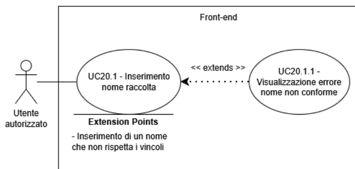
Figure 35: UC20.1 - Inserimento nome raccolta
