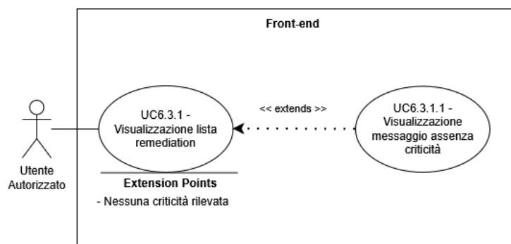
Figure 15: UC6.3.1 - Visualizzazione lista remediation
