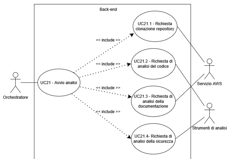
Figure 37: UC21 - Avvio analisi
