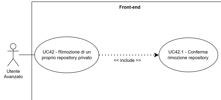
Figure 51: UC42 - Rimozione di un proprio repository privato
