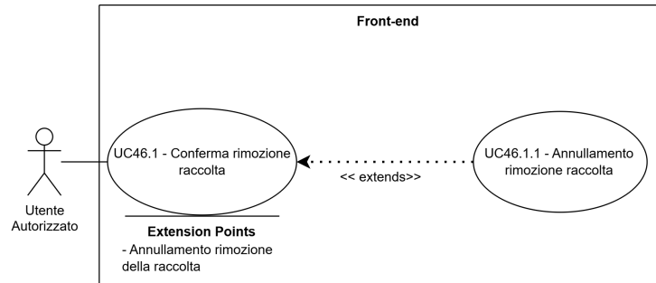
Figure 58: UC46 - Conferma rimozione raccolta
