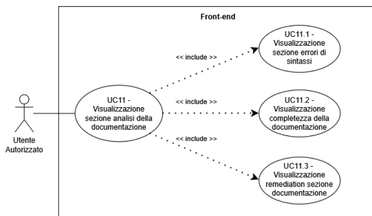
Figure 21: UC11 - Visualizzazione sezione analisi della documentazione
