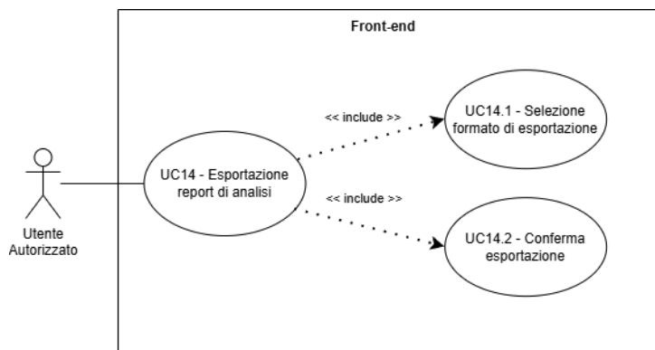
Figure 24: UC14 - Esportazione report di analisi
