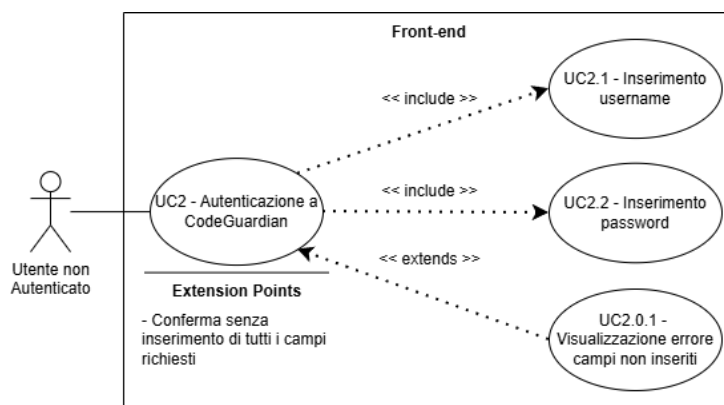
Figure 5: UC2 - Autenticazione
