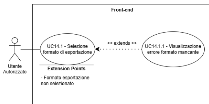
Figure 25: UC14.1 - Selezione formato di esportazione
