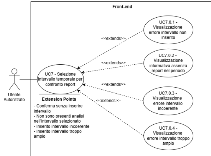
Figure 16: UC7 - Selezione intervallo temporale per confronto report
