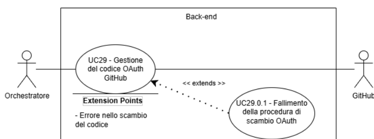
Figure 44: UC29 - Gestione del codice OAuth GitHub
