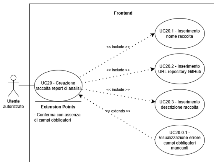
Figure 34: UC20 - Creazione raccolta report di analisi
