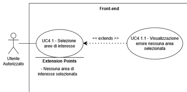
Figure 9: UC4.1 - Selezione aree di interesse
