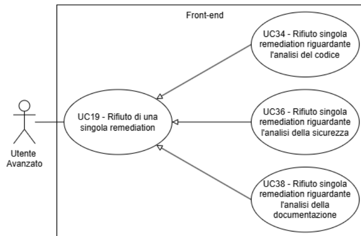
Figure 33: UC19 - Rifiuto singola remediation generica
