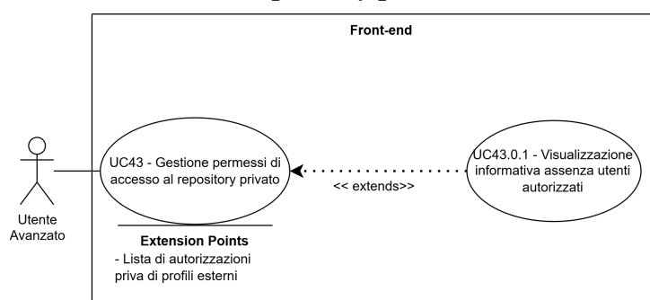
Figure 53: UC43 - Gestione permessi di accesso al repository privato
