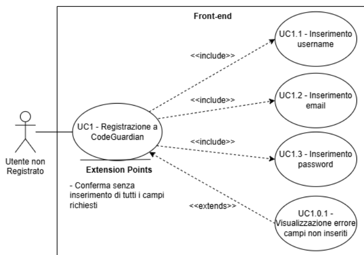
Figure 1: UC1 - Registrazione
