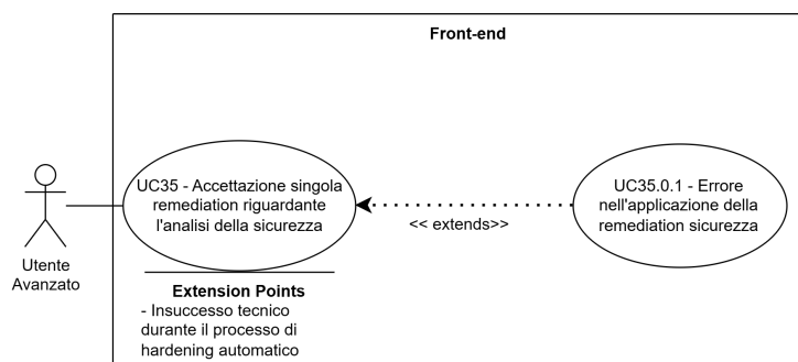
Figure 46: UC35 - Accettazione singola remediation riguardante l'analisi della sicurezza
